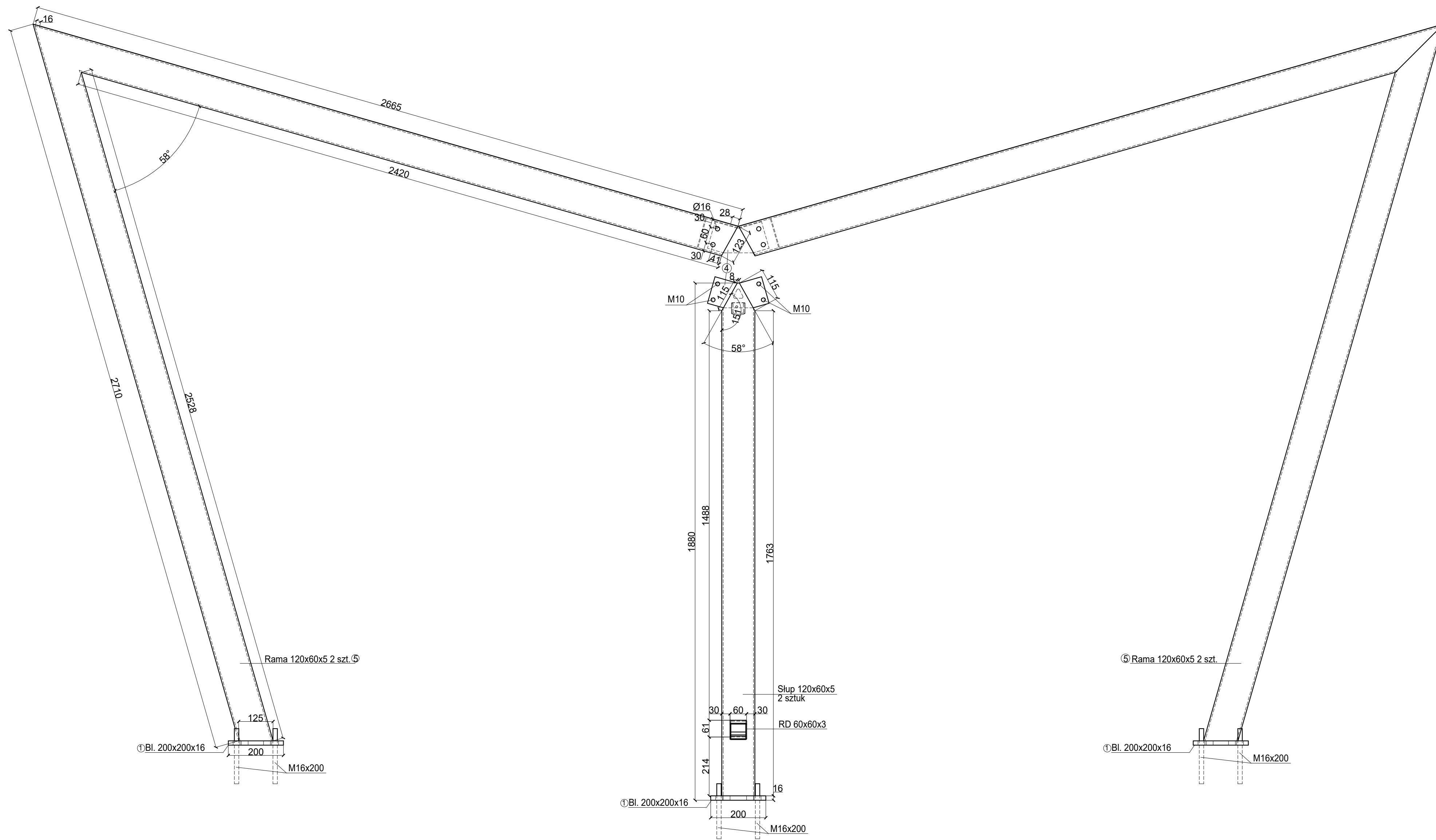
RYŚ. WIATY 1C - SCHEMAT MONTAŻOWY, WYKROJE BL.
